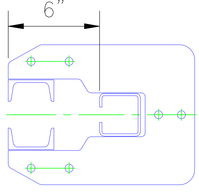
VIEW "A-A" SCALE: 3"=1'-0"
