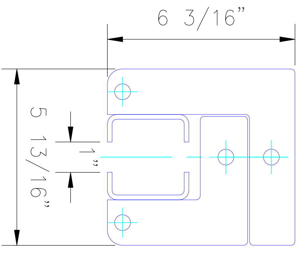
SECTION VIEW "A-A" SCALE: 6"=1'-0"
